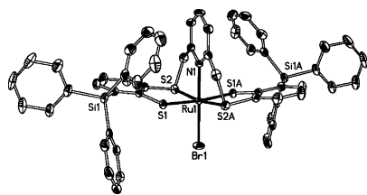
Figure 3. ORTEP diagram of 4 (50% probability ellipsoids; H atoms and solvent molecules omitted). Selected distances [ \text{Å} ] and angles [ ^\circ ]: \text{Ru1}-\text{N1} 2.055(3), \text{Ru1}-\text{Br1} 2.5239(4), \text{Ru1}-\text{S1} 2.3153(6), \text{Ru1}-\text{S2} 2.3101(6), \text{N1}-\text{Ru1}-\text{Br1} 180.000(1), \text{N1}-\text{Ru1}-\text{S1} 86.90(2), \text{N1}-\text{Ru1}-\text{S2} 84.66(2), \text{S1}-\text{Ru1}-\text{S2} 88.14(2), \text{S1}-\text{Ru1}-\text{S1A} 173.79(3), \text{S2}-\text{Ru1}-\text{S2A} 169.33(3).
